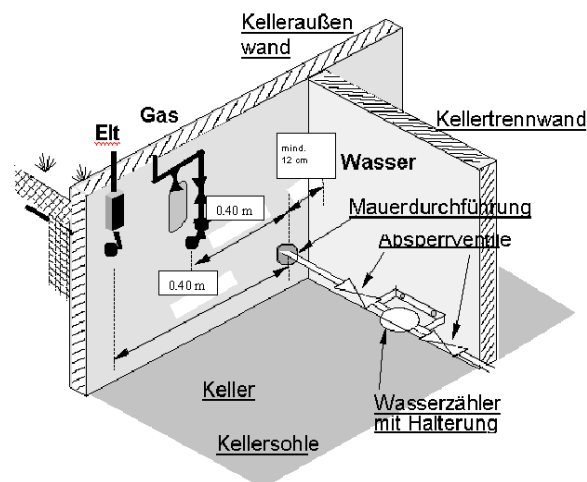
Beispiel für die Anordnung der Hausanschlussleitung im Hausanschlussraum nach DIN 18012
